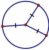
Radii
